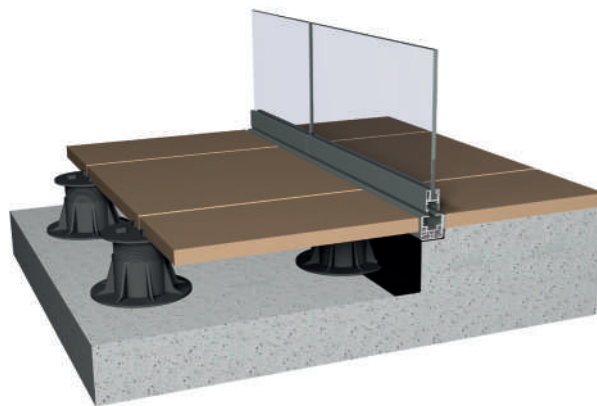
Connessione a pavimento
